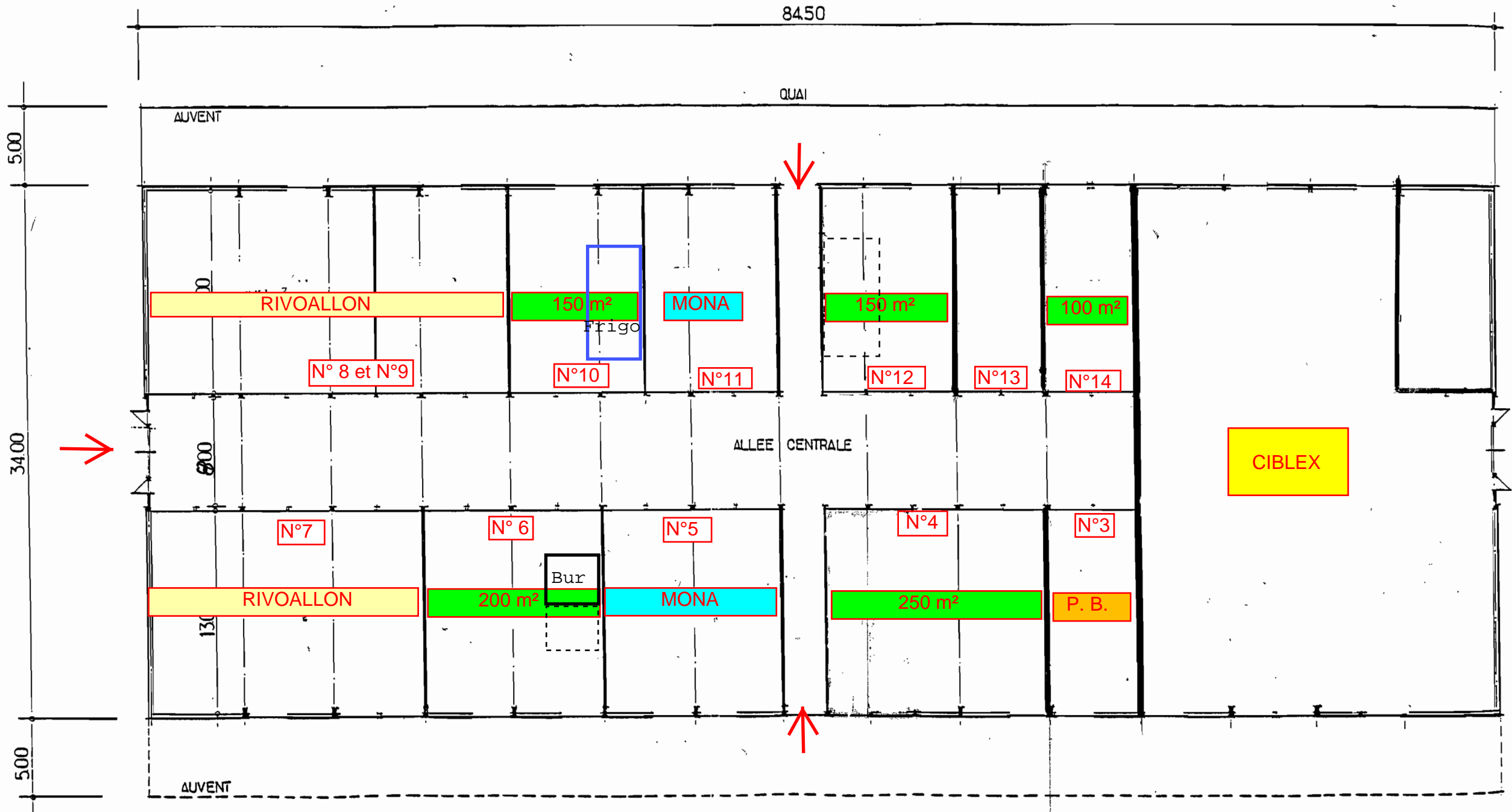
PLAN D'ENSEMBLE
